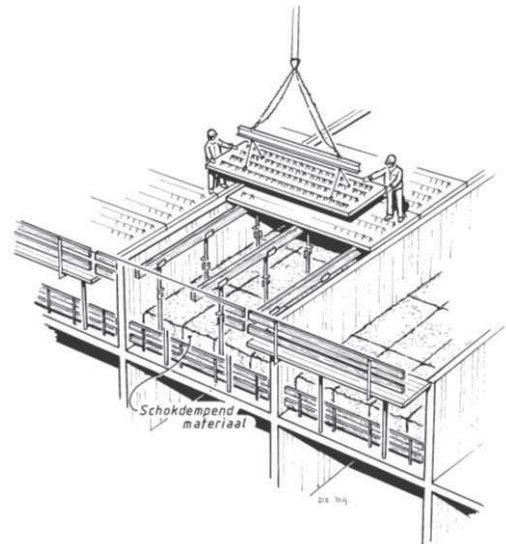
Figuur 7 Schokdempend materiaal op de onder- liggende vloer als beveiliging/bescherming aan het legfont
